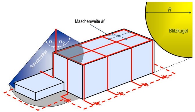
Verfahren für die Auslegung von Fangeinrichtungen: Schutzwinkel, Masche, Blitzkugel (Quelle: VDE)
