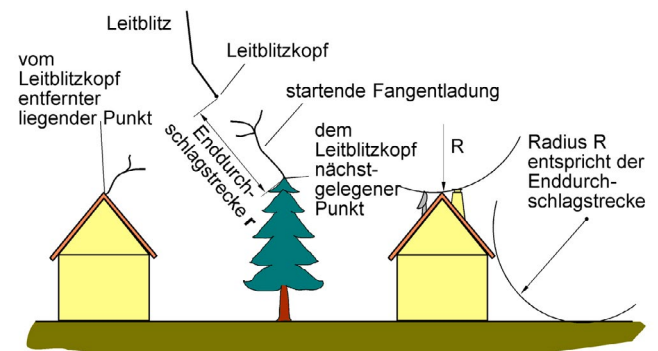
Das elektro-geometrische Modell: startende Fangentladung, die die Einschlagstelle festlegt (Quelle: VDE)
