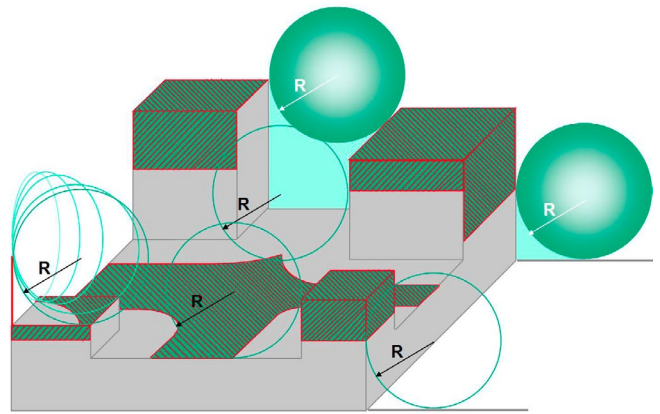
Blitzkugel-Verfahren bei einem Gebäudekomplex mit stark gegliederter Oberfläche: Die schraffierten Flächen sind mögliche Einschlagstellen des Blitzes, die durch Fangeinrichtungen geschützt werden müssen. (Quelle: VDE)
