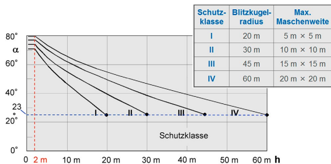
Schutzwinkel, Blitzkugel-Radius und Maschenweite von Fangeinrichtungen in Abhängigkeit von der Blitzschutzklasse (Quelle: VDE)
