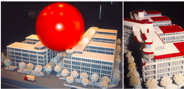
DAS-Verwaltungsgebäude: Modell mit Blitzkugel der Schutzklasse I (links); blitzeinschlaggefährdete Bereiche rot gefärbt (rechts) (Quelle: VDE)
