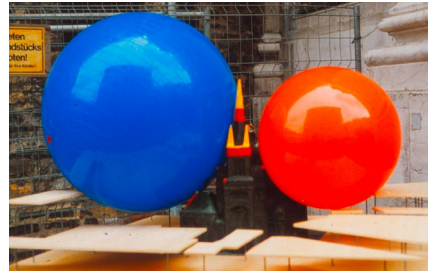
Aachener Dom: Modell mit Umgebung und Blitzkugeln der Schutzklasse II und III (Quelle: VDE)
