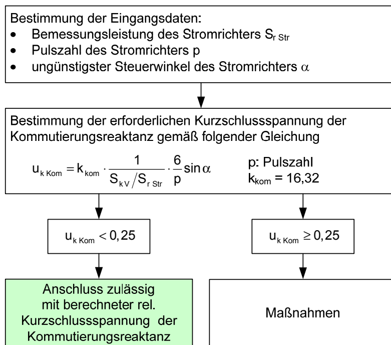
Abb. B4-2: Schema zur detaillierten Beurteilung nach Stufe 2
