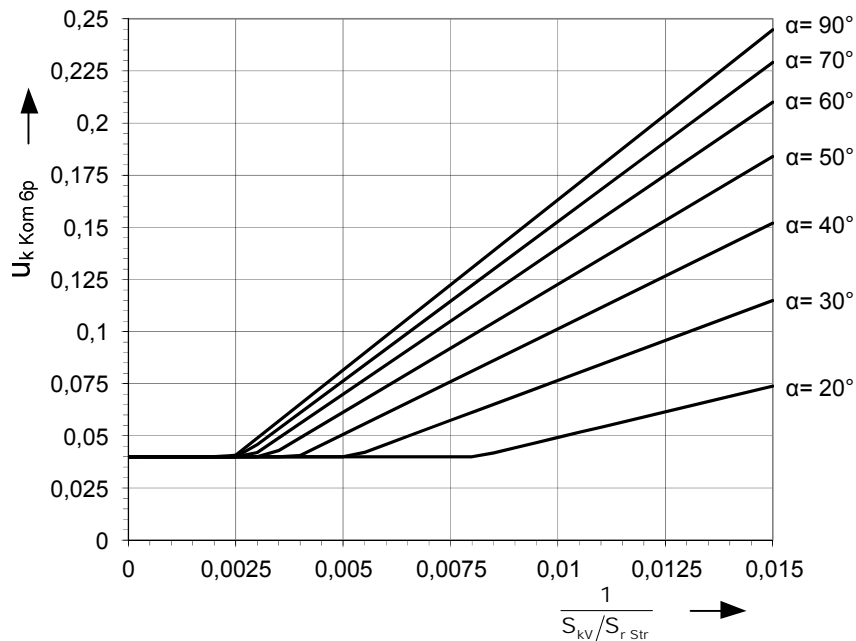
Abb. B4-3: Erforderliche relative Kurzschlussspannung u_{k,Kom} der Kommutierungsreaktanz X_{Kom} in Abhängigkeit vom Verhältnis 1/(S_{kv}/S_{r,Str}) für verschiedene Steuerwinkel für 6-pulsige Stromrichter
