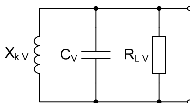
Abb. B3-1: vereinfachtes Ersatzschaltbild zur Modellierung der ersten Parallelresonanzstelle
