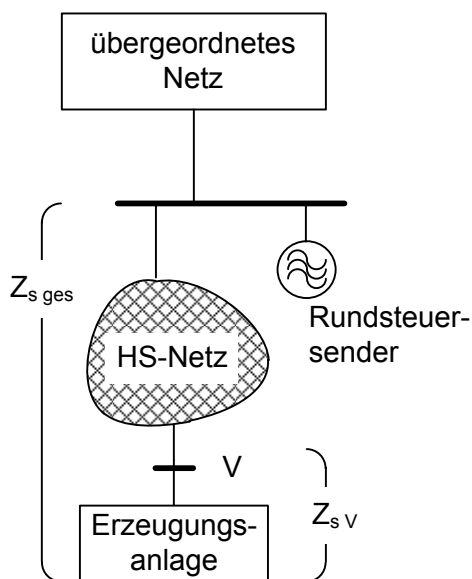
Abb. C7-1: Allgemeines Ersatzschaltbild
