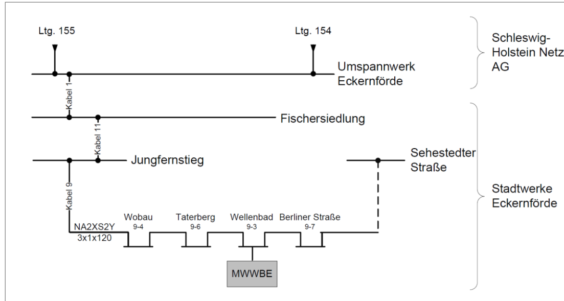
MS-Netzinfrastruktur und Netzanschluss des MWWBE, Quelle: Buchmüller/Gehlert/Schütt, Schwimmbäder als zuschaltbare Lasten, 2017, S. 34
