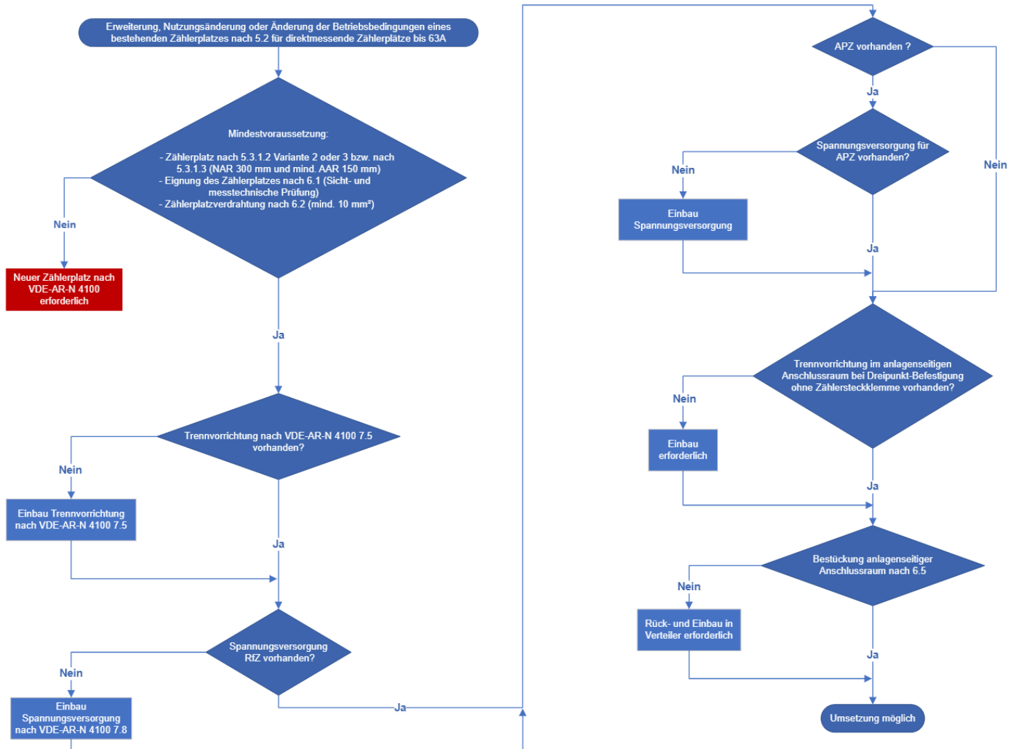
Bild 7 - Prozessdarstellung
